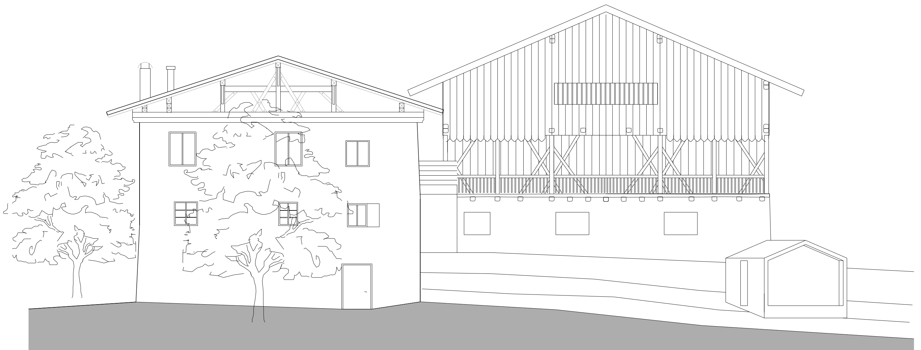
Ansicht Süd
